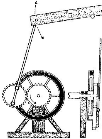
ワットの蒸気機関に使われた遊星歯車(18世紀)
