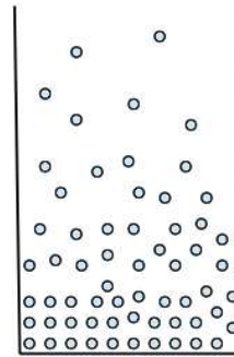
図2 微粒子の沈降分布の模式図
